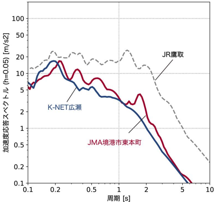
加速度応答スペクトル Sa
