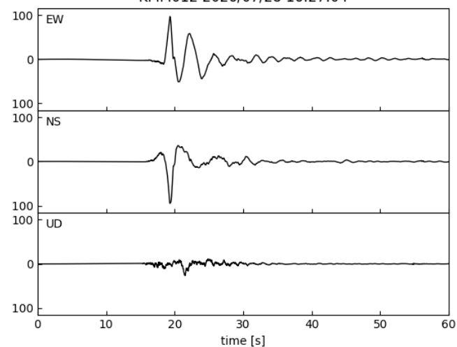
K-NET八代 速度波形 KMM012 2026/07/28 16:27:04
