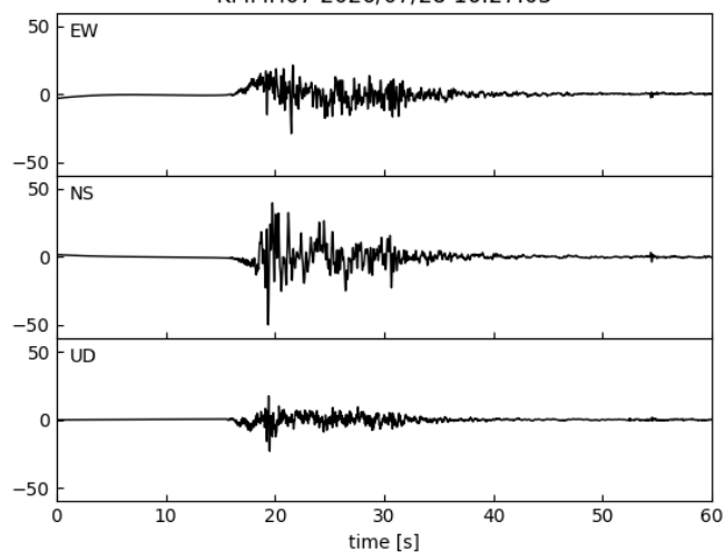
KiK-net三角 速度波形 KMMH07 2026/07/28 16:27:03
